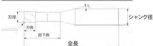
超硬ロングネックスクエアエンドミルの各部位
