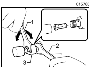
1. 17 号扳手 2. 10 号扳手 3. 筒夹螺母
