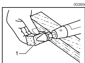
1. 磨石
